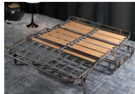
Standardbeslag: Gurte und Gitterrost Abbildung: alternativer Beslag mit Gurten und Lattenunterfederung
